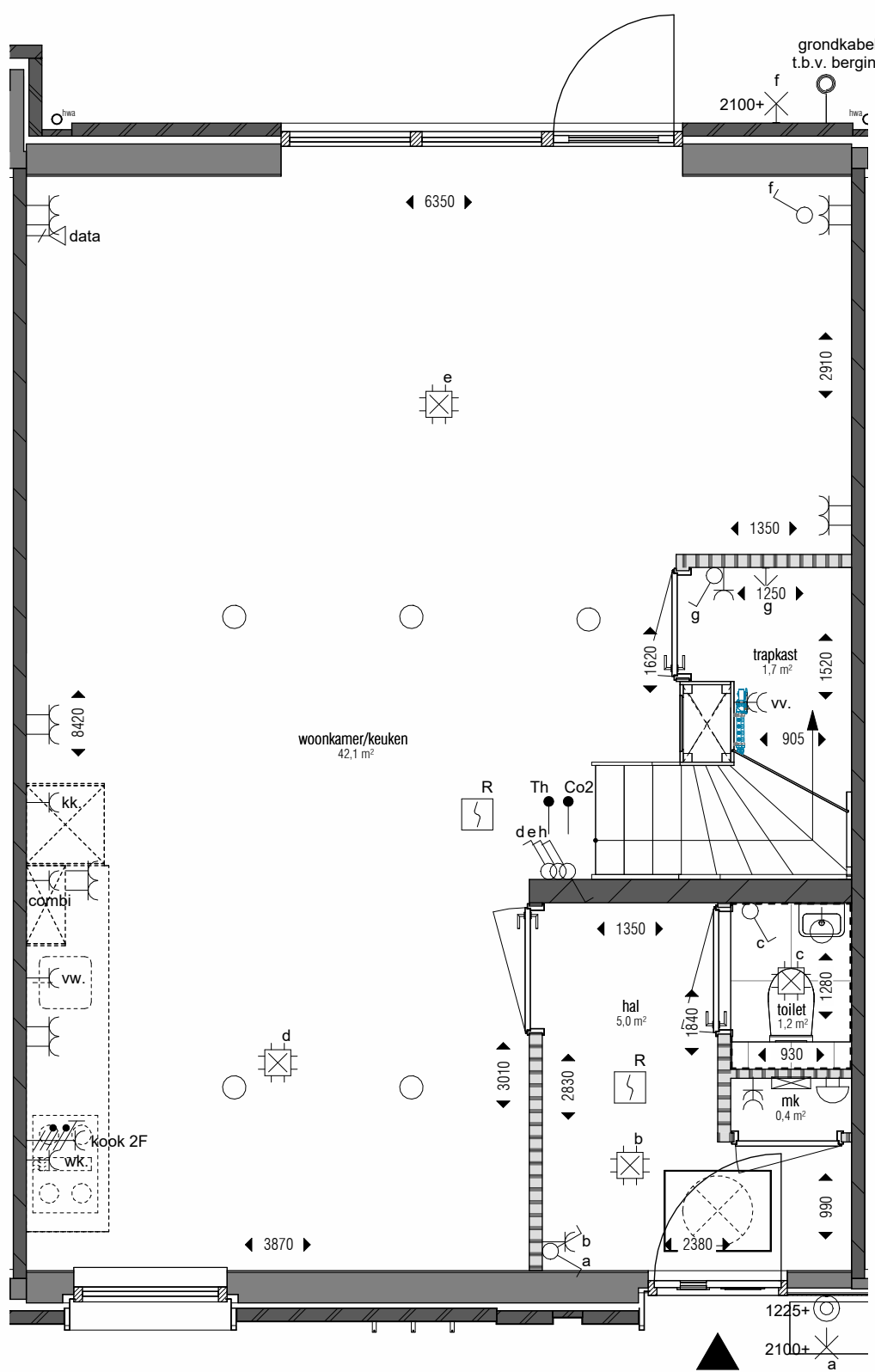
begane grond 1:50
