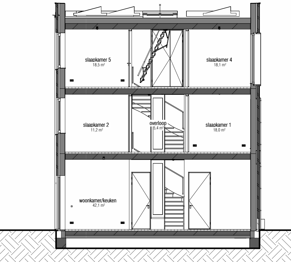
doorsnede 1:100
