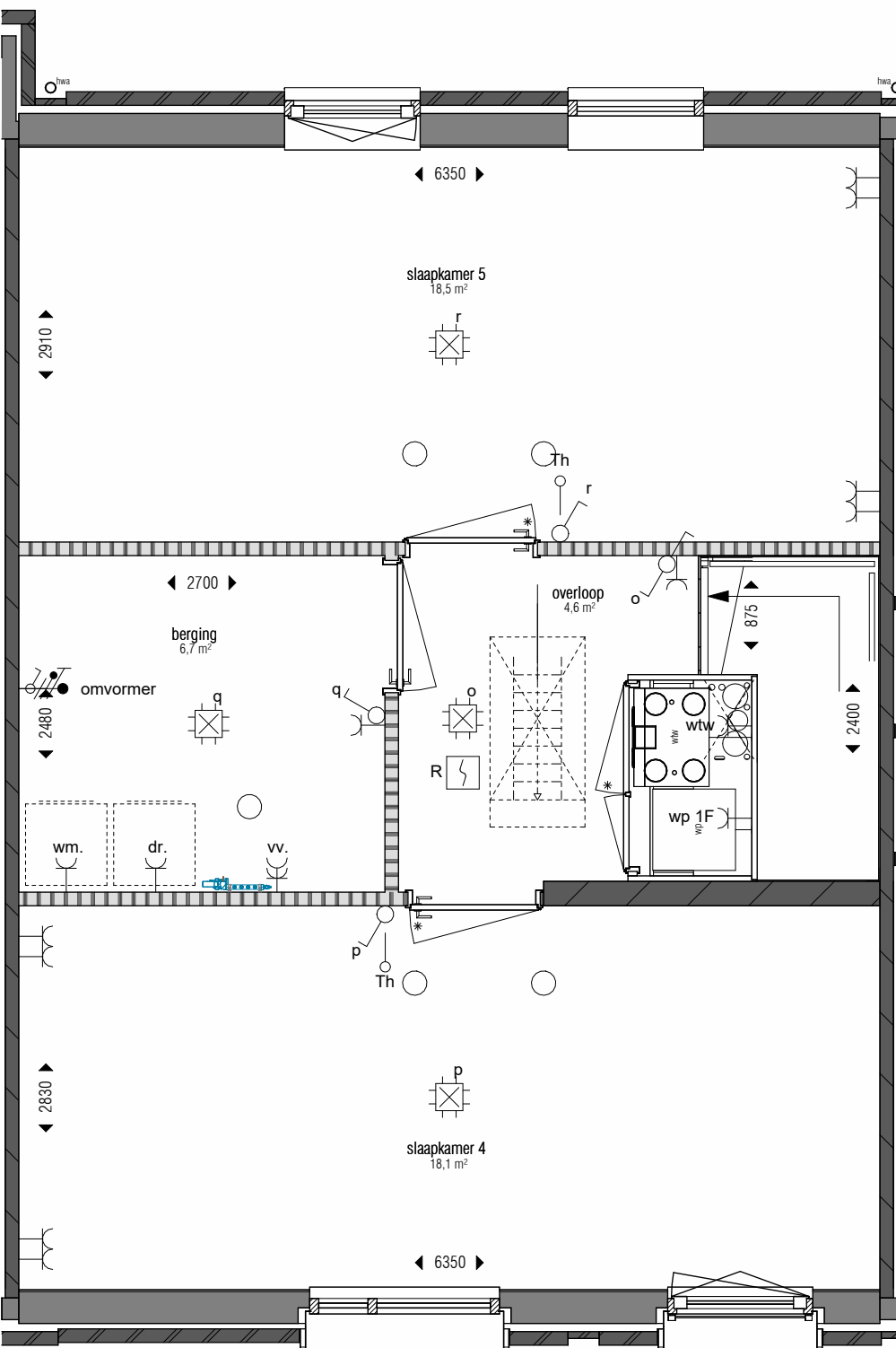
tweede verdieping 1:50
