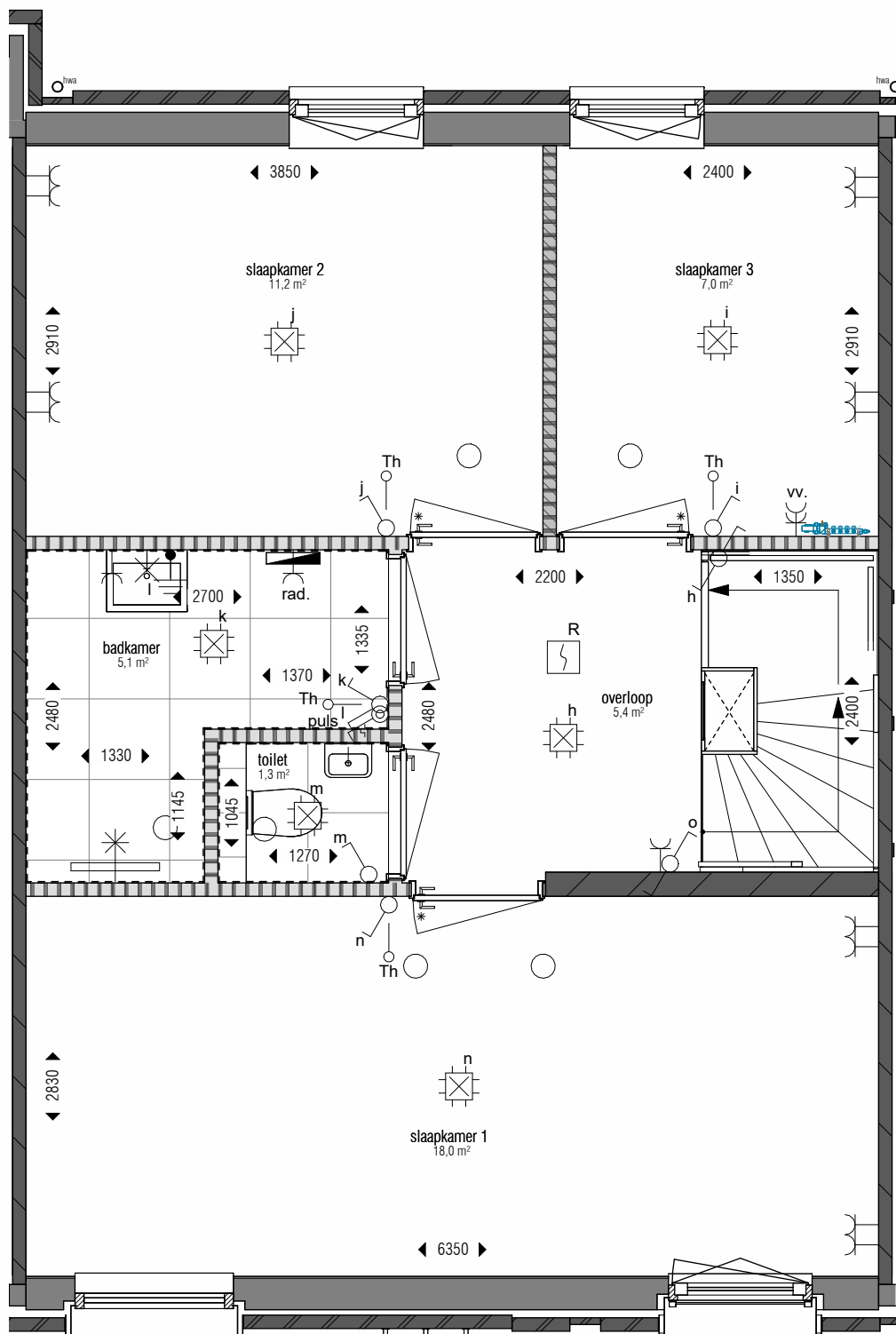
eerste verdieping 1:50
